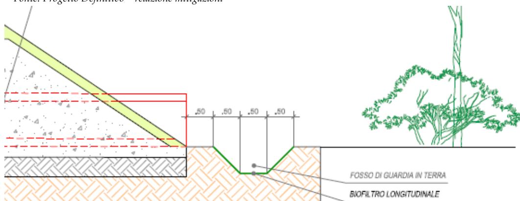
Figura 59 – Biofiltri longitudinali Fonte: Progetto Definitivo – relazione mitigazioni
