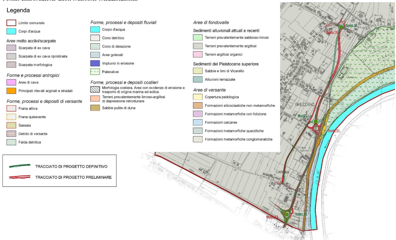
Figura 48 – Sovrapposizione alla Carta geomorfologica (Nodi 10-11-12) Fonte: Elaborazione Geol. Massimo Mezzananza
