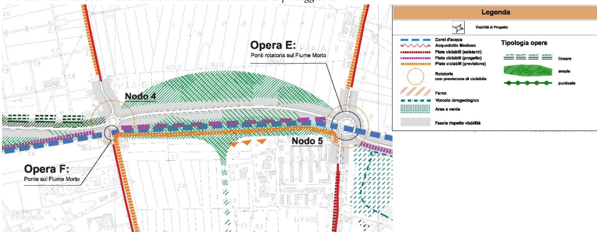
Figura 92 – Opere di mitigazione nel tratto Nodi 4-5 Fonte: Elaborato G08 - Elaborazione tridimensionale dell'ambito paesaggistico
