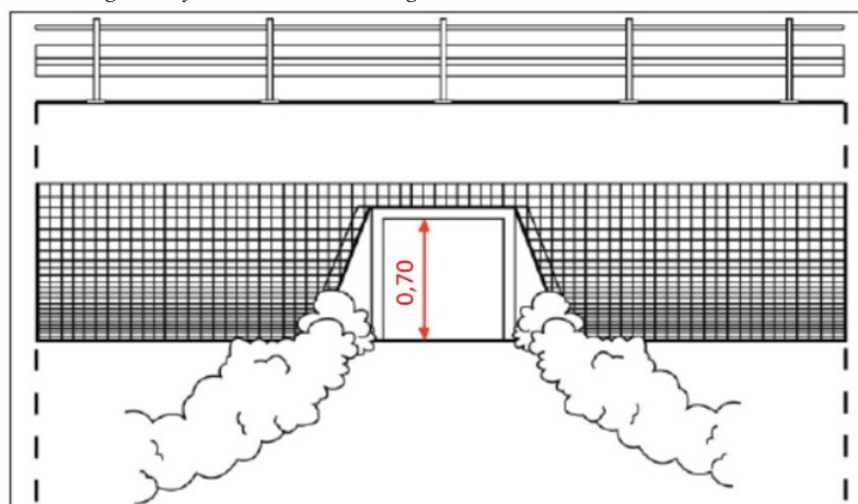
Figura 61 – Sottopassi per anfibi Fonte: Progetto Definitivo – relazione mitigazioni
