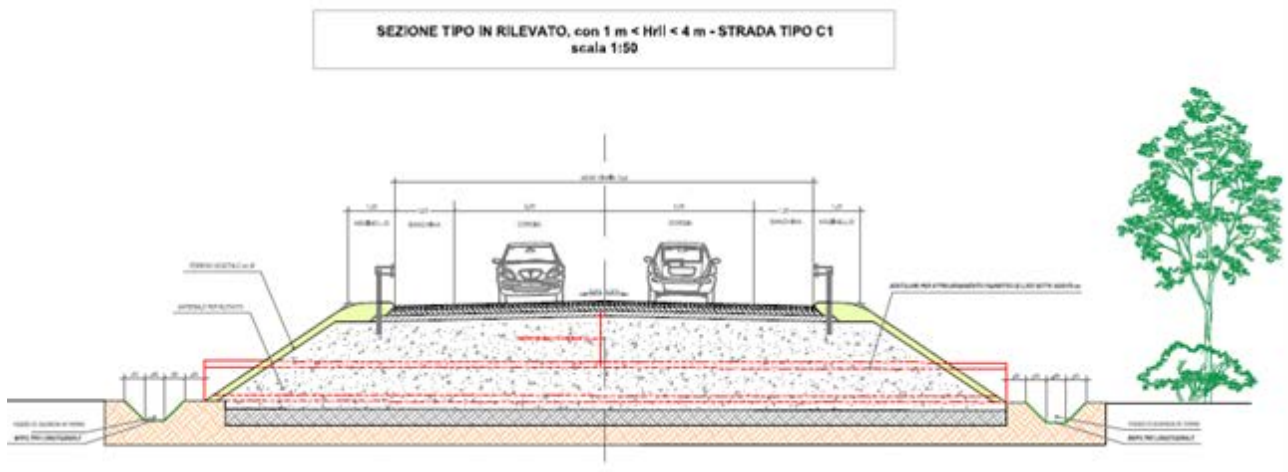
Figura 103 – Sezione tipo nel tratto tra i nodi 1 e 2 – Progetto Definitivo: eliminazione del terrapieno “tipo dune” Fonte: Relazione di Variante
