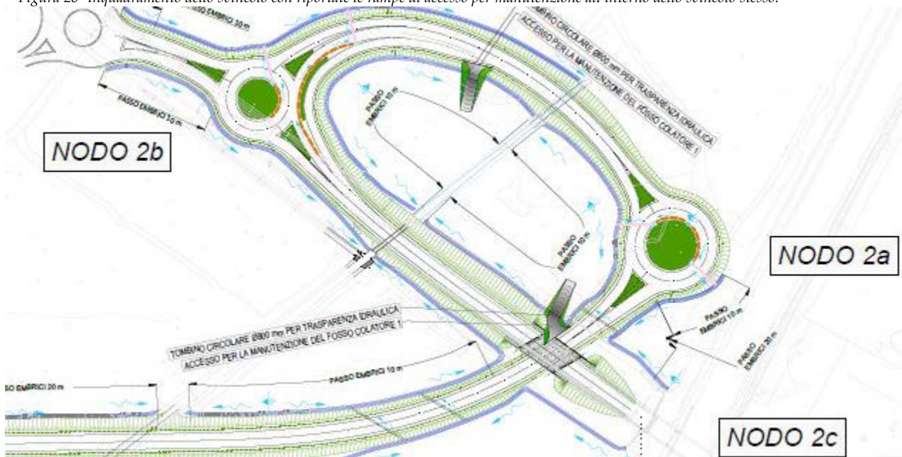
Figura 28- Inquadratura dello svincolo con riportate le rampe di accesso per manutenzione all'interno dello svincolo stesso.
