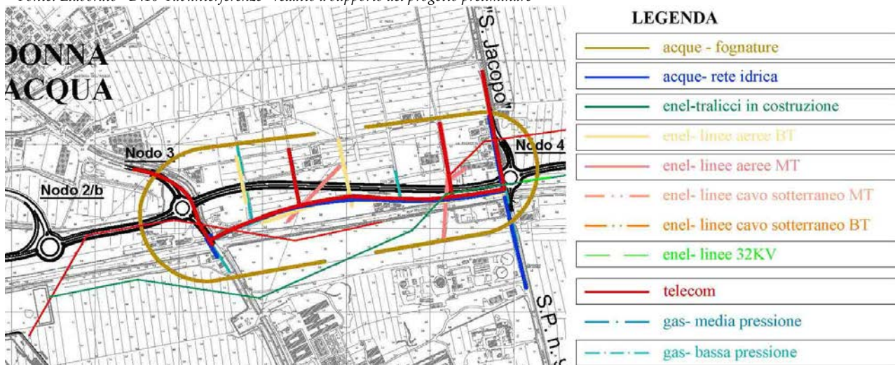
Figura 19 – Interferenze tra il nodo 2 ed il nodo 4
