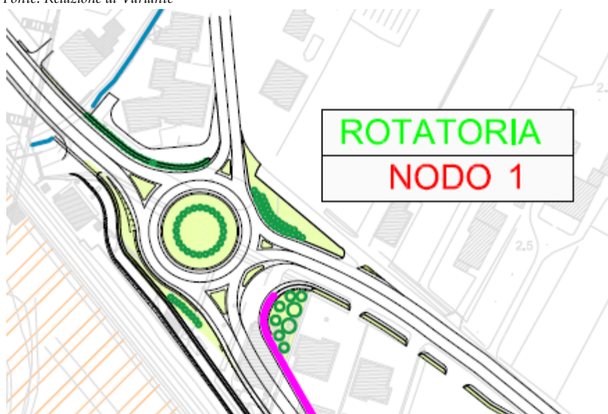
Figura 99 - Nodo 1 particolare delle mitigazioni in planimetria
