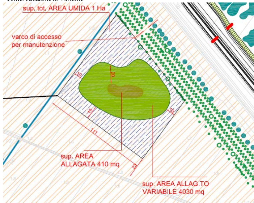
Figura 65 - Area umida in progetto - Pianta Fonte: Relazione di Variante
