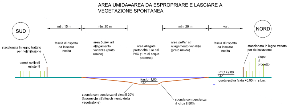
Figura 66 - Area umida in progetto - Sezione Fonte: Relazione di Variante
