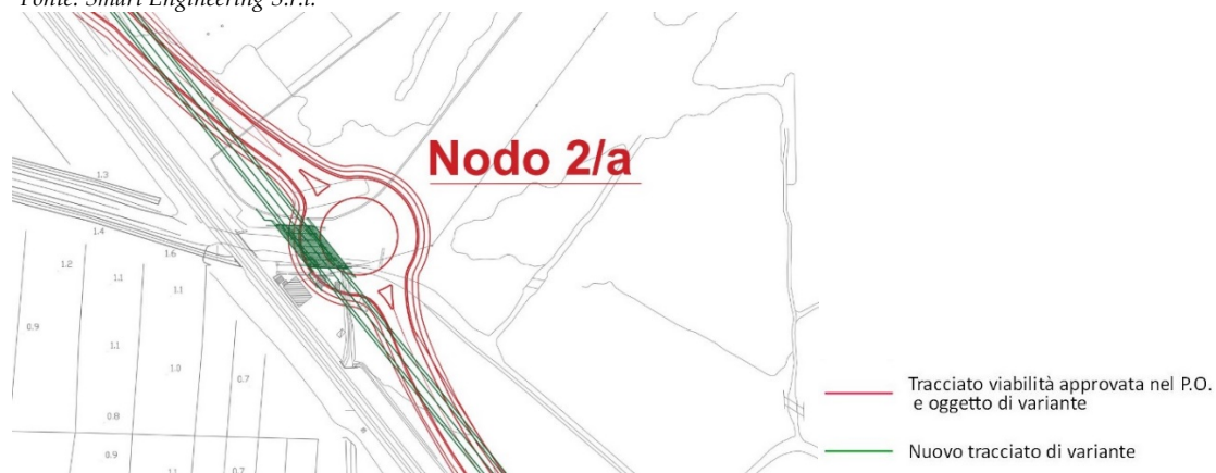
Figura 12 – EX Nodo 2/a Fonte: Smart Engineering S.r.l.
