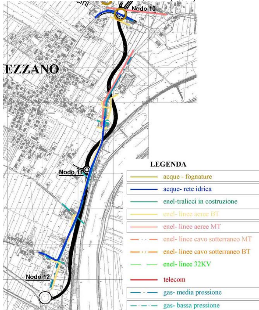
Figura 21 – Interferenze tra il nodo 10 ed il nodo 12
