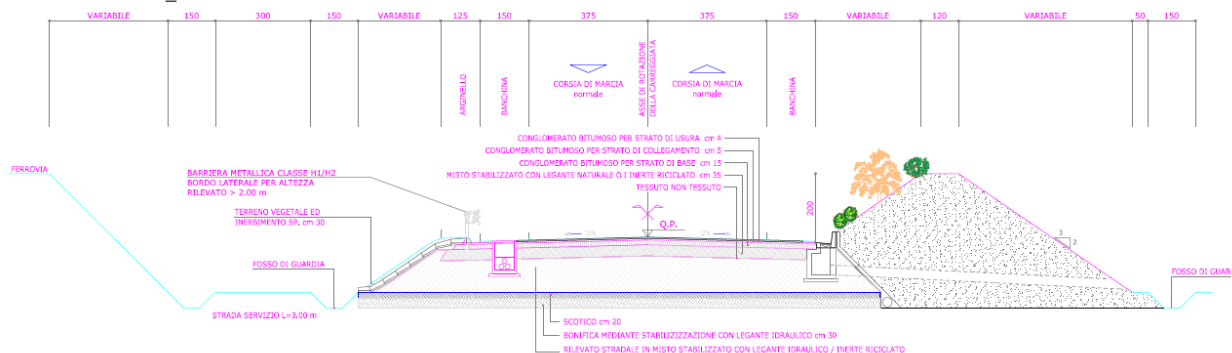
Figura 44- Sezione stradale tratto 1-2 con ipotesi terrapieno lato opposto ferrovia Fonte: "D.08.02_SEZIONI TIPO E PARTICOLARI COSTRUTTIVI"
