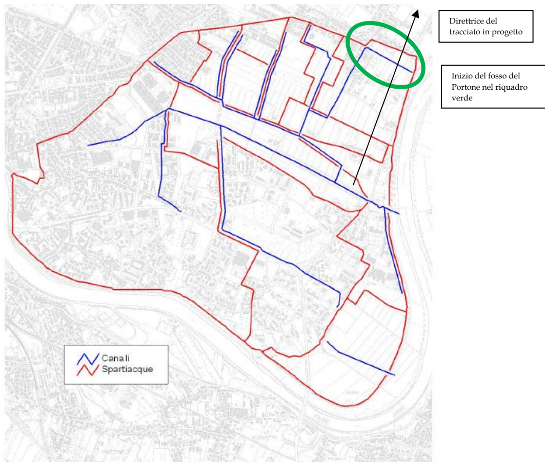
Figura 4-1 – Canali e bacini idrografici nello stato di progetto
