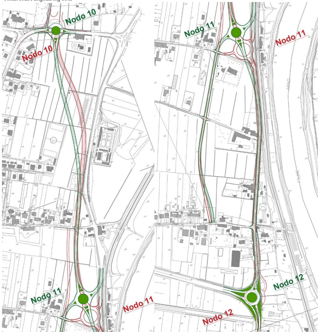
Figura 17 – Tratta Nodi 10-11 e Nodi 11- 12 Fonte: Smart Engineering S.r.l.
