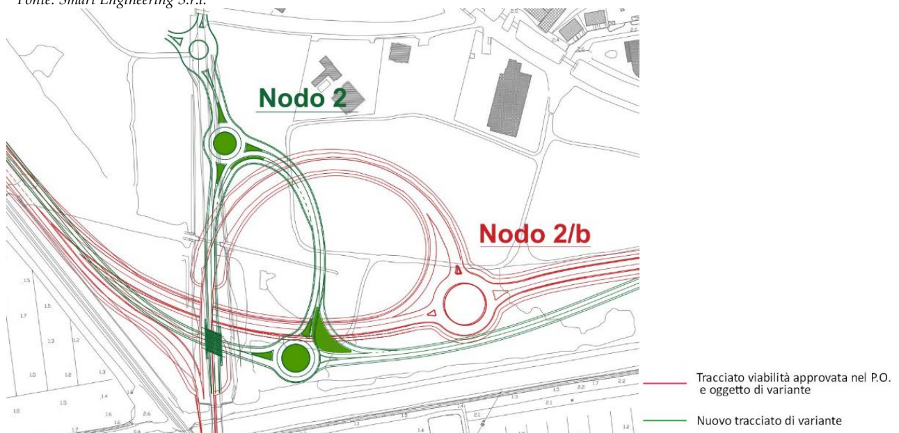
Figura 13 – Nodo 2 Fonte: Smart Engineering S.r.l.
