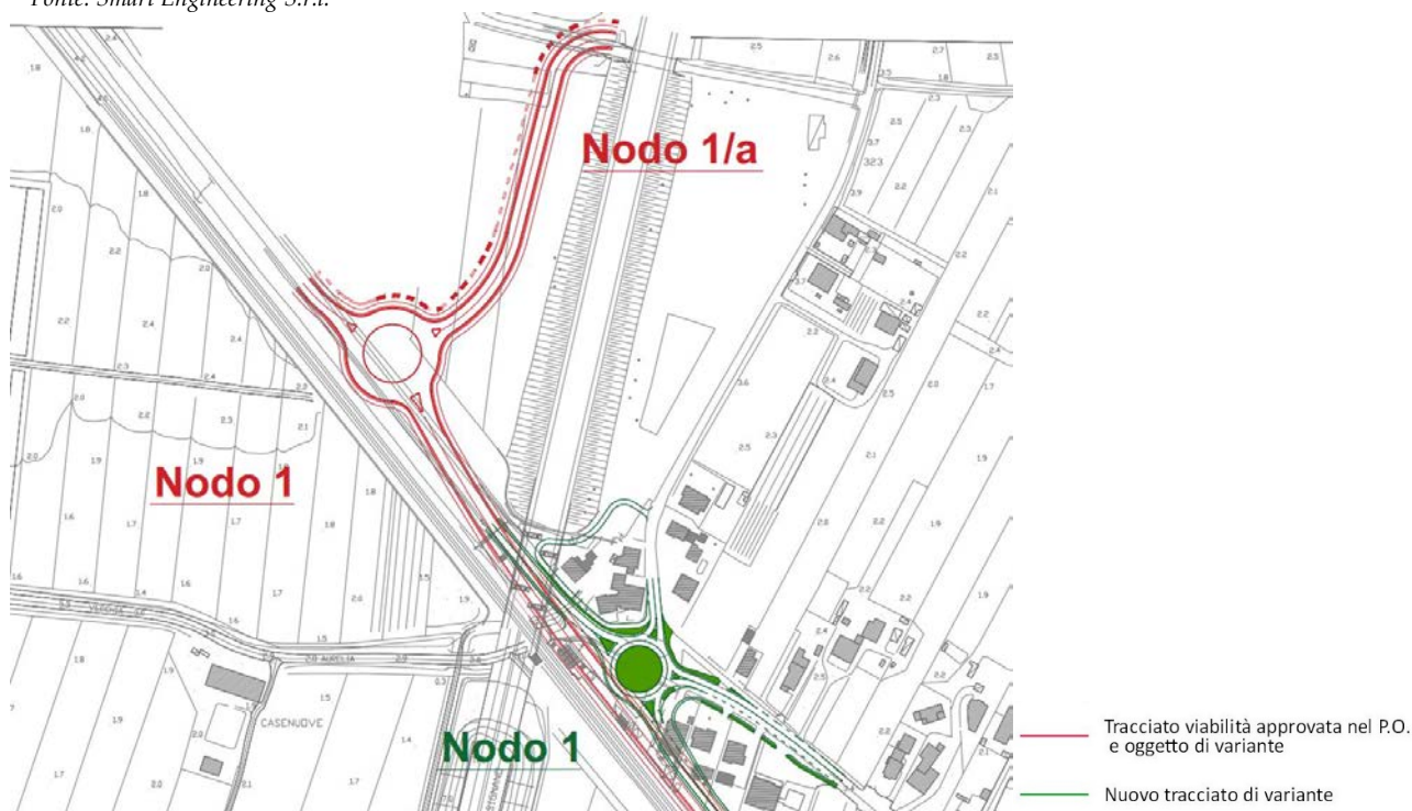
Figura 11 – Nodo 1 Fonte: Smart Engineering S.r.l.
