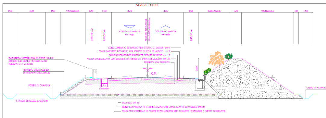
Figura 102 - Sezione tipo nel tratto tra i nodi 1 e 2 - Progetto Preliminare: terrapieno "tipo dune"
