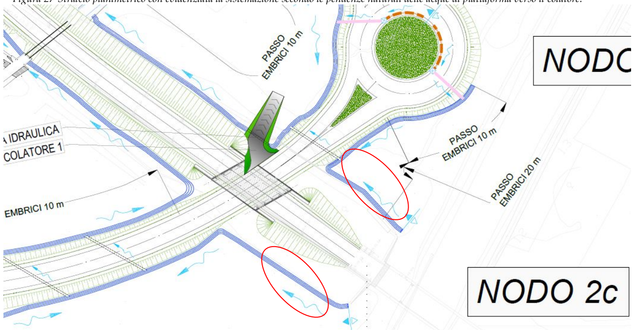
Figura 27-Stralcio planimetrico con evidenziata la sistemazione secondo le pendenze naturali delle acque di piattaforma verso il colatore.
