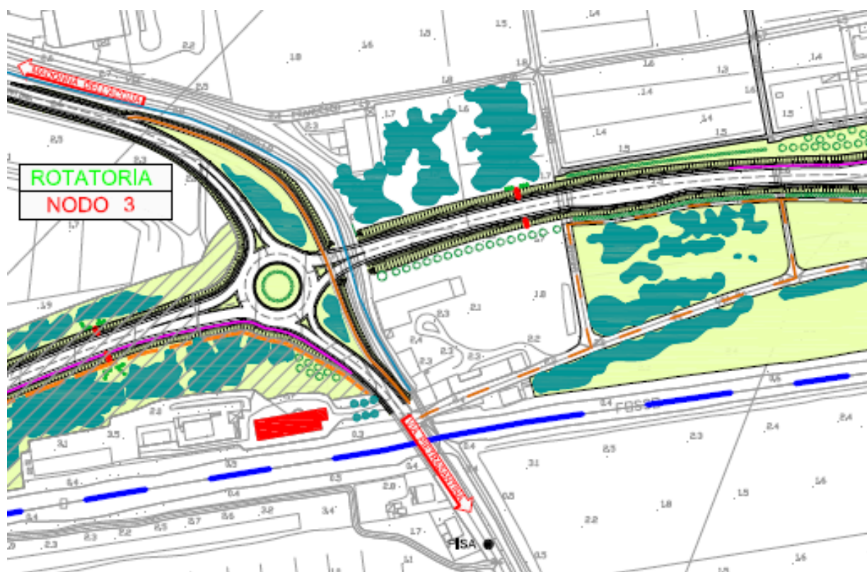
Figura 105 - Planimetria nei pressi del nodo 3 Fonte: Relazione di Variante
